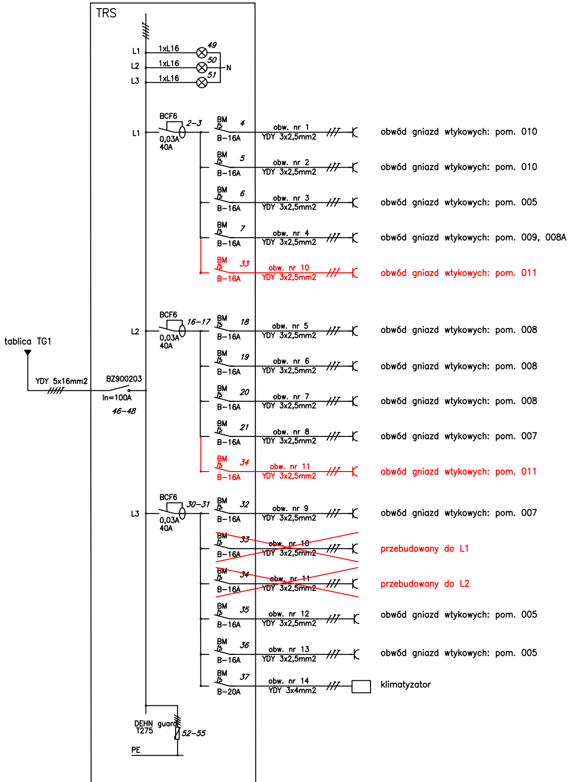
obudowa tablicy bezpiecznikowej TRS wnętkowa 4x14, II klasa izolacji typ BK070004 4x14 SCHRACK
