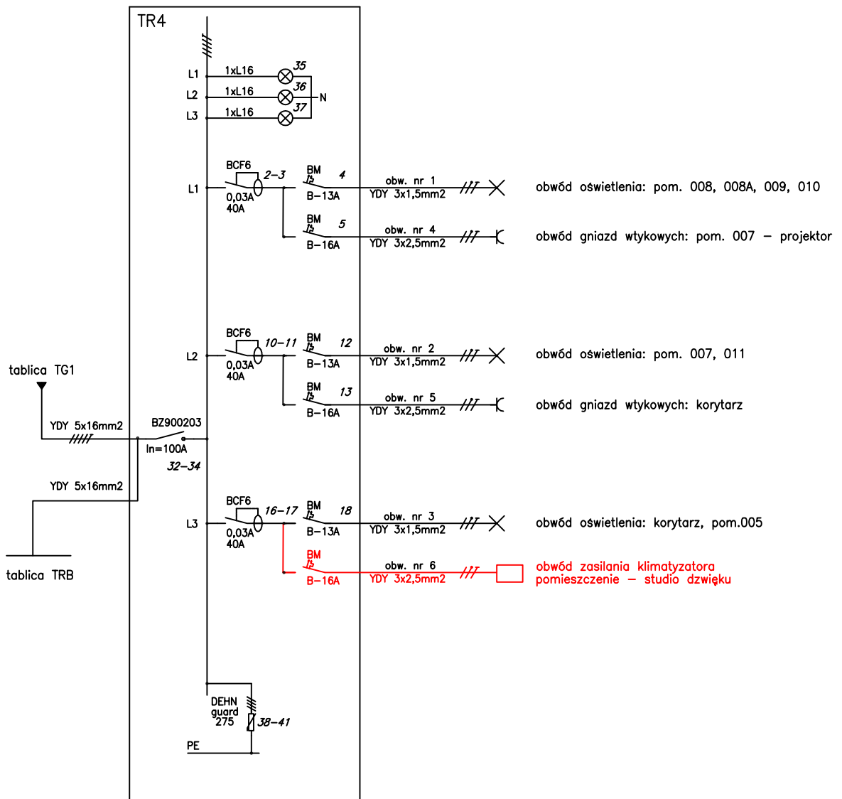
obudowa tablicy bezpiecznikowej TR4 wnętkowa 3x14, II klasa izolacji typ BK070004 3x14 SCHRACK
