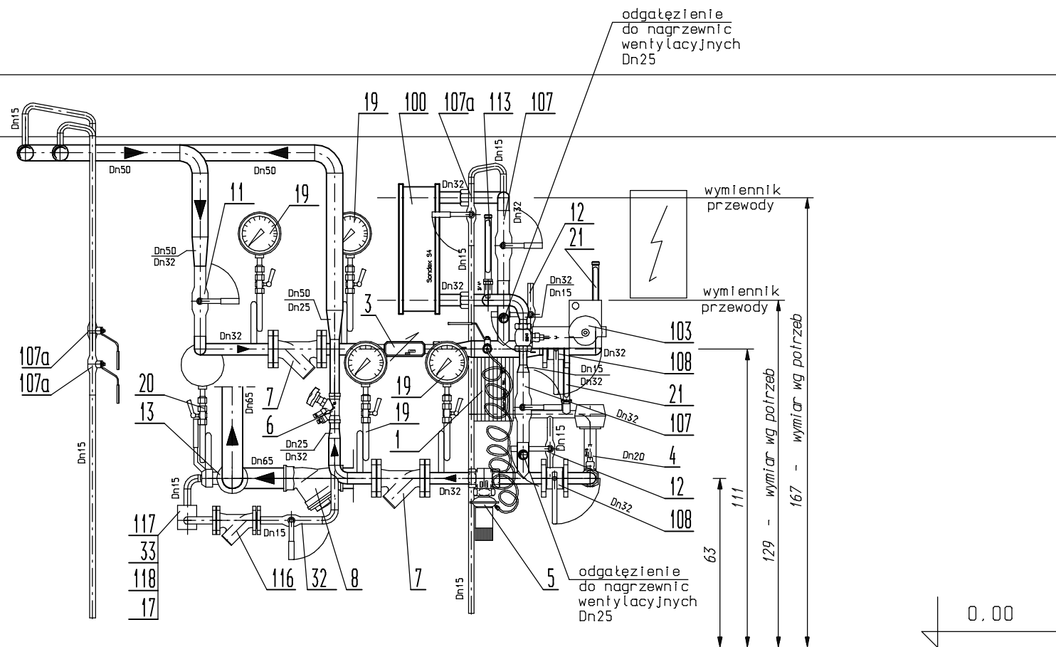
PRZEKRÓJ A-A
