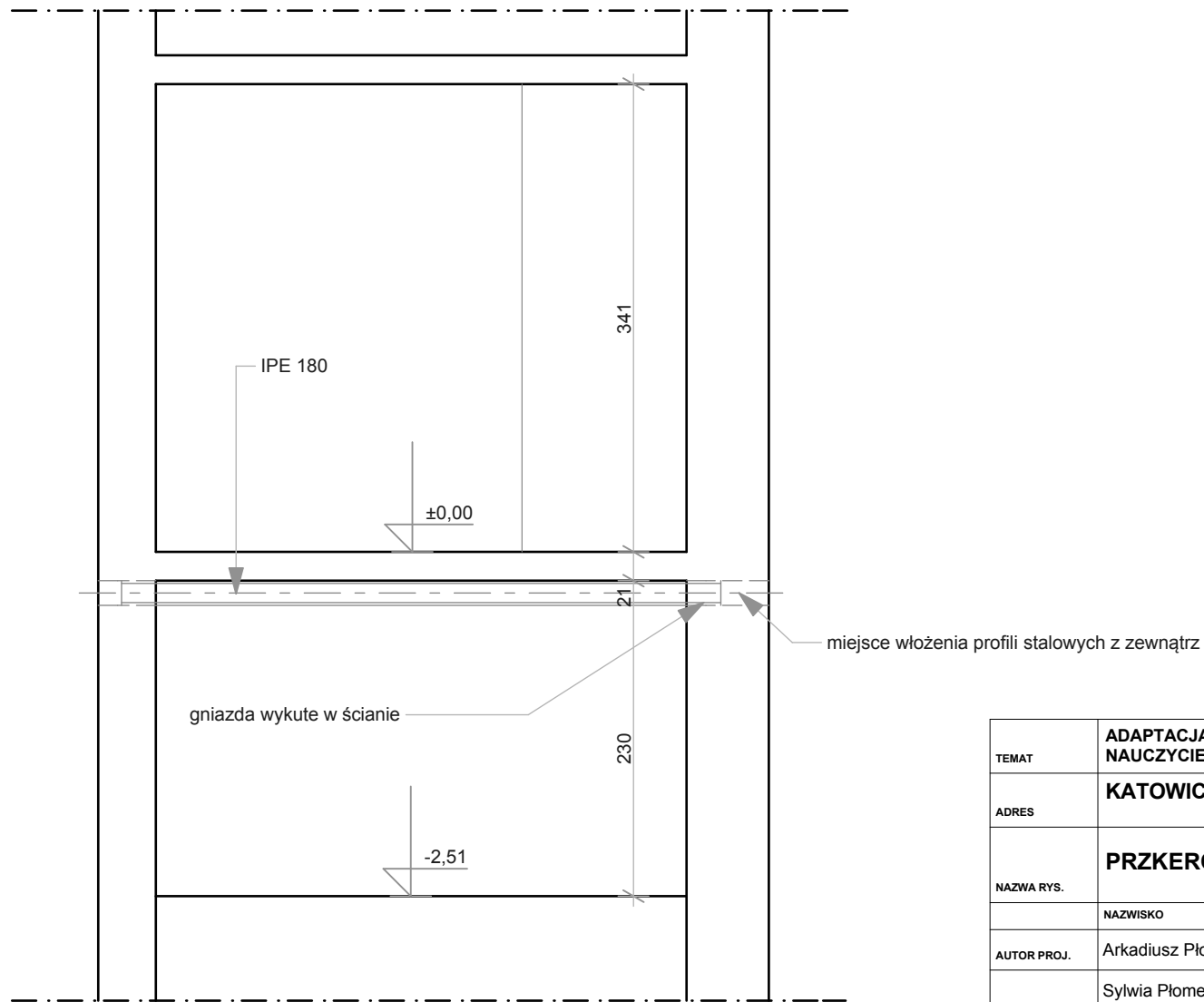
PRZEKRÓJ - PROJEKT
