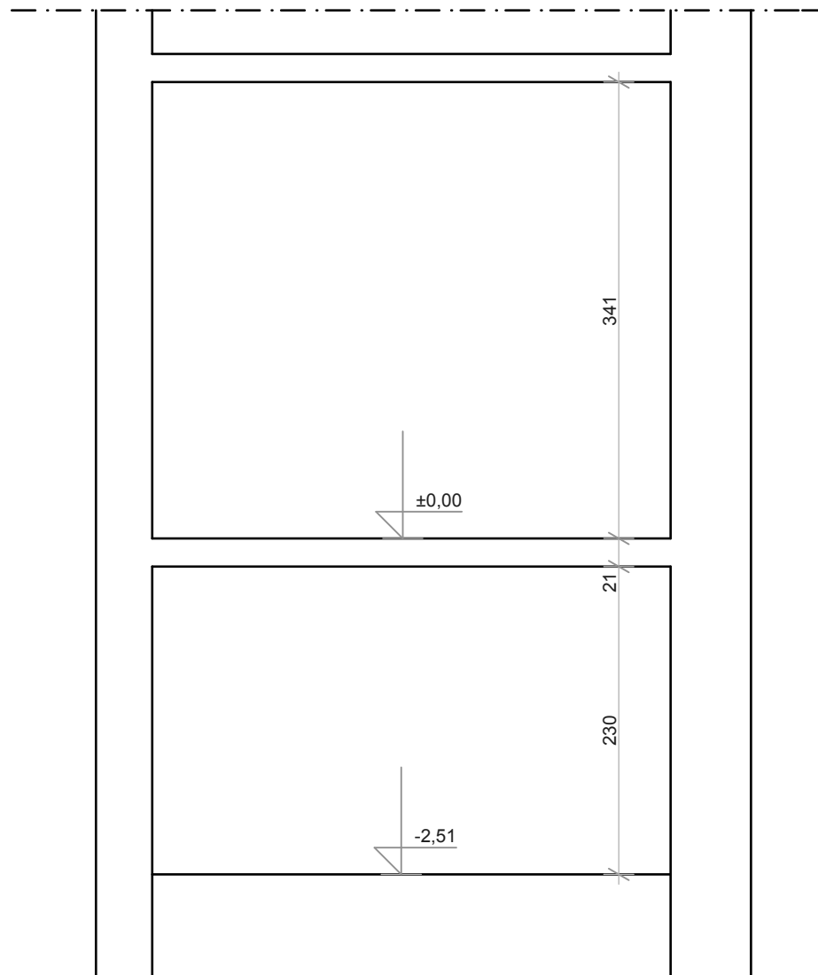
PRZEKRÓJ - INWENTARYZACJA
