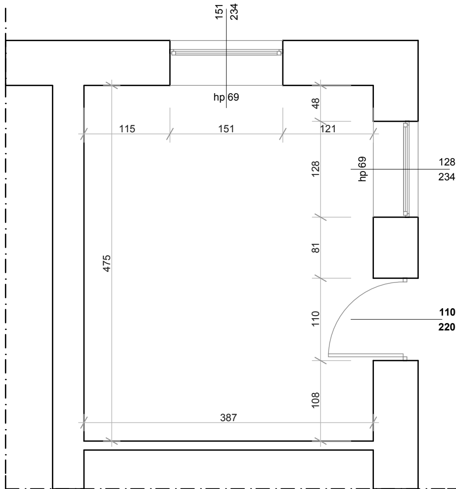
RZUT PARTERU - INWENTARYZACJA
