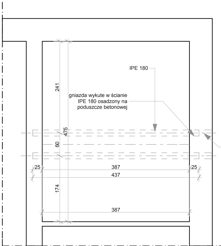
RZUT PIWNIC - PROJEKT
