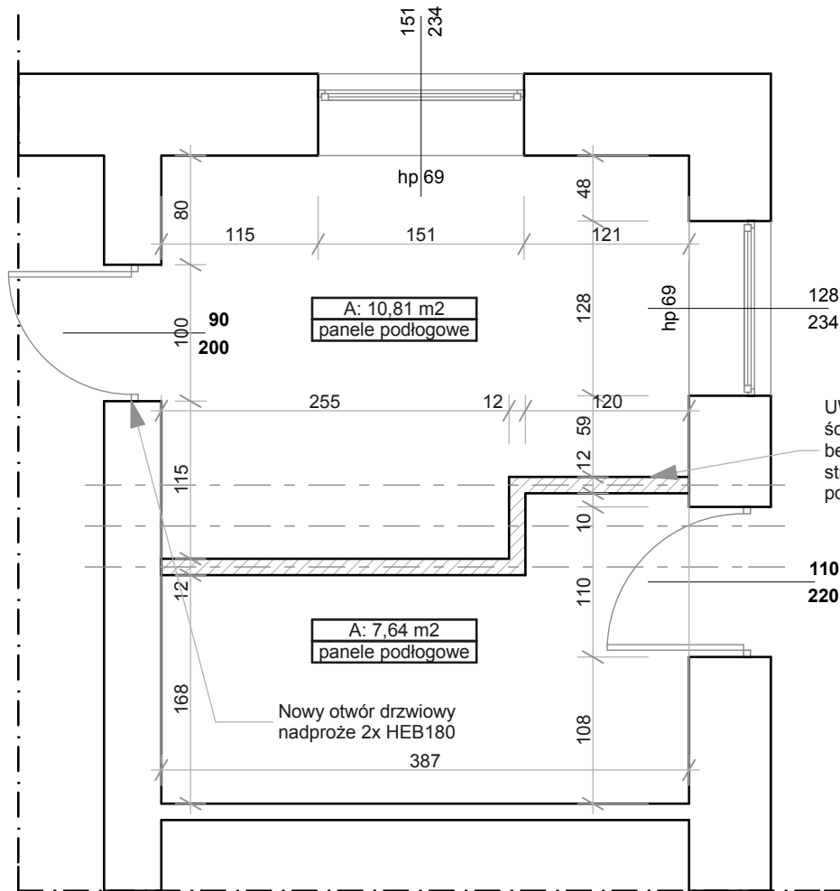
RZUT PARTERU - PROJEKT
