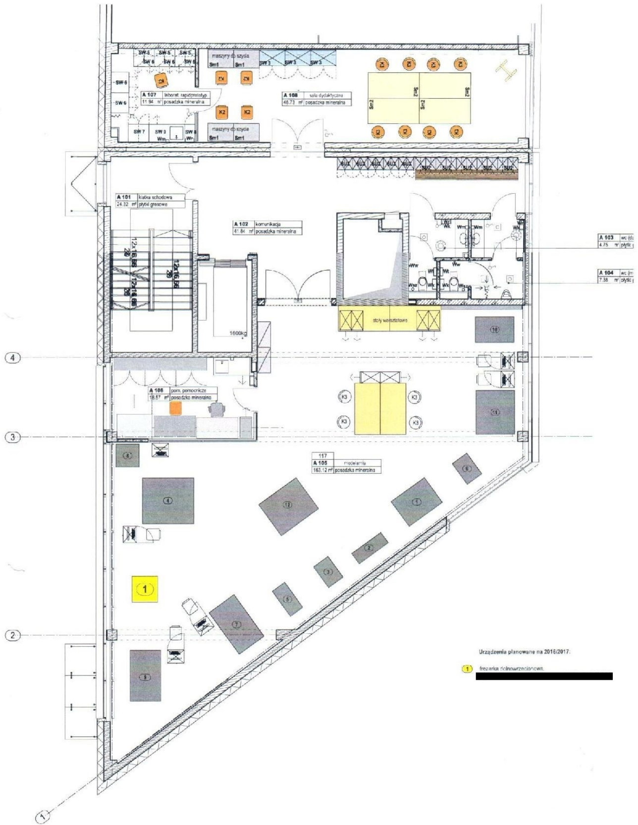
UKŁAD URZĄDZEŃ I WYPOSAŻENIA MODELARNI POZ. 1 aktualizacja 30.05.2016
